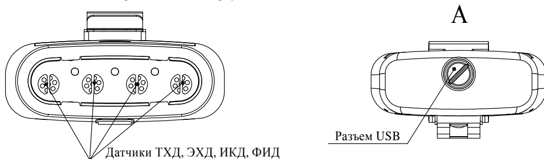
Газоанализатор со снятым побудителем расхода или блоком поверочным. Вид сверху
