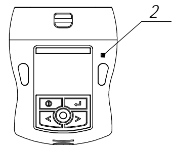
е) диффузионный отбор пробы (температура окружающего воздуха от минус 30 до плюс 45 °С, побудитель расхода (блок для ручного отбора пробы) поз.1 (б) - снят)
